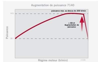
Case IH FPT 8,7 litres sur moissonneuses-batteuses 6140 et 7140
